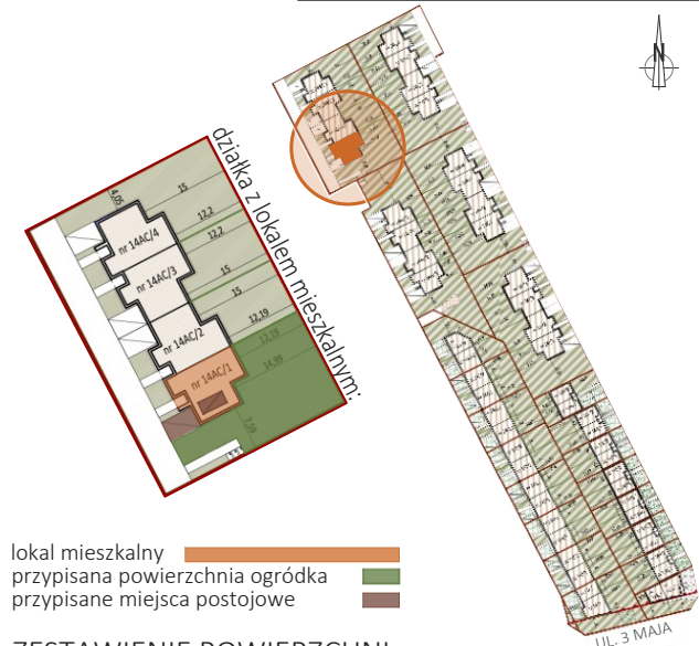
PLAN INWESTYCJI
